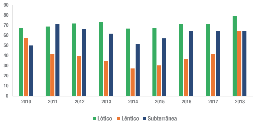
Proporção de corpos hídricos lóticos, lânticos e subterrâneos com boa qualidade da água - 2010-2018 (%)
