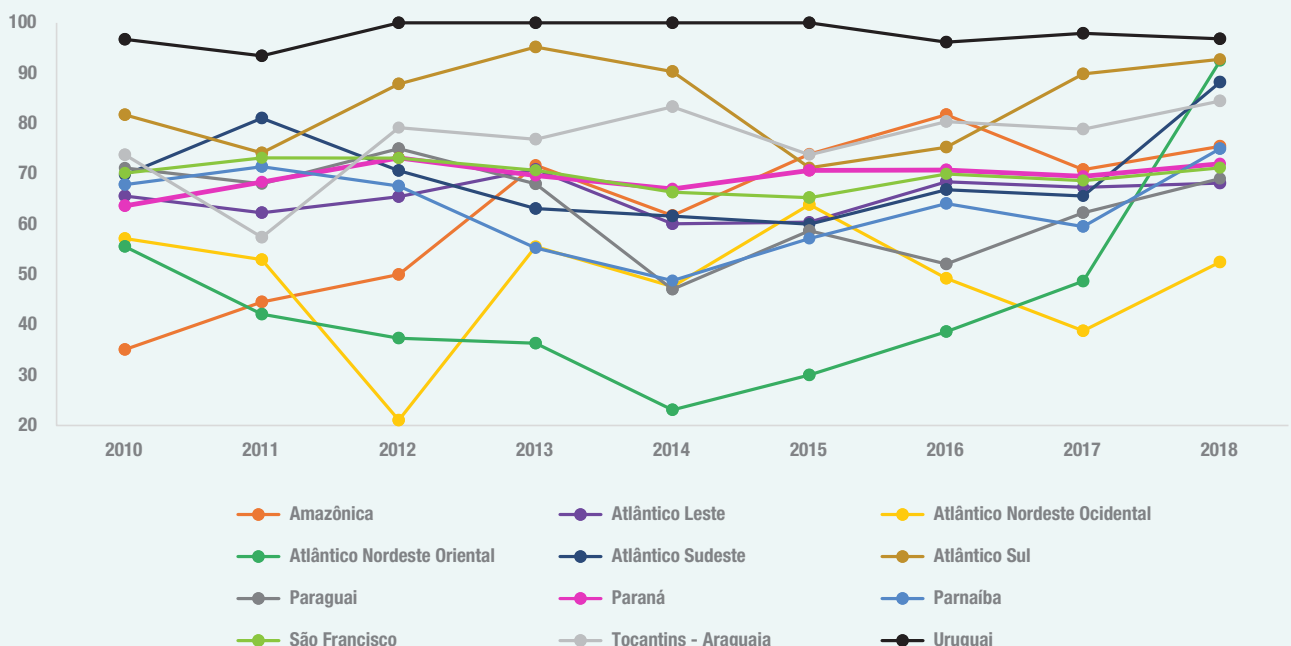
Proporção de corpos hídricos com boa qualidade da água por Região Hidrográfica 2010-2018 (%)
