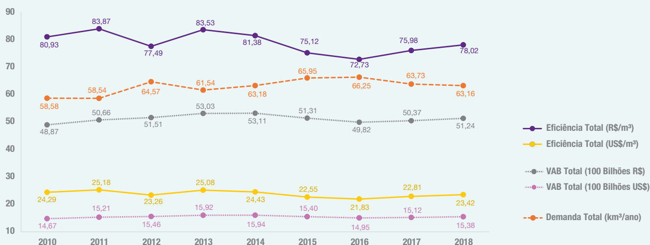
Evolução da eficiência do uso da água no Brasil no período 2010 - 2018
