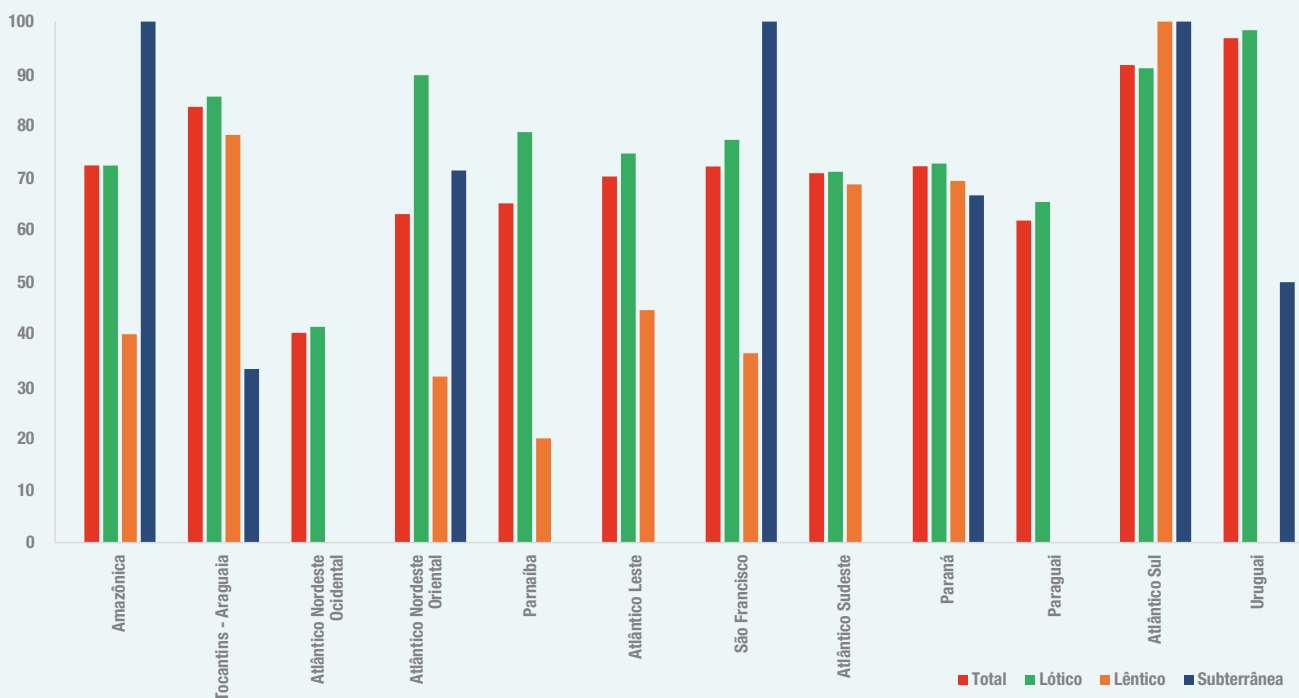
Proporção de corpos hídricos com boa qualidade da água por tipologia e Região Hidrográfica - 2017-2018 (%)
